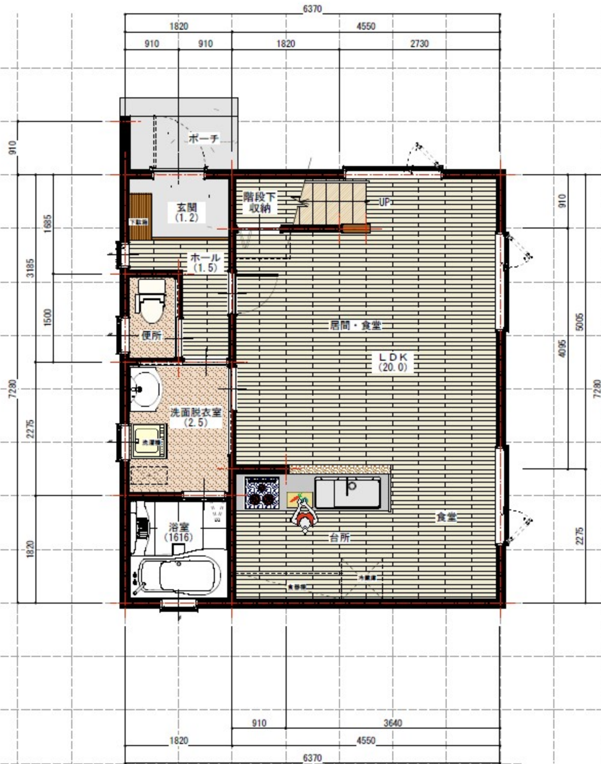
1階平面図 S=1:50
